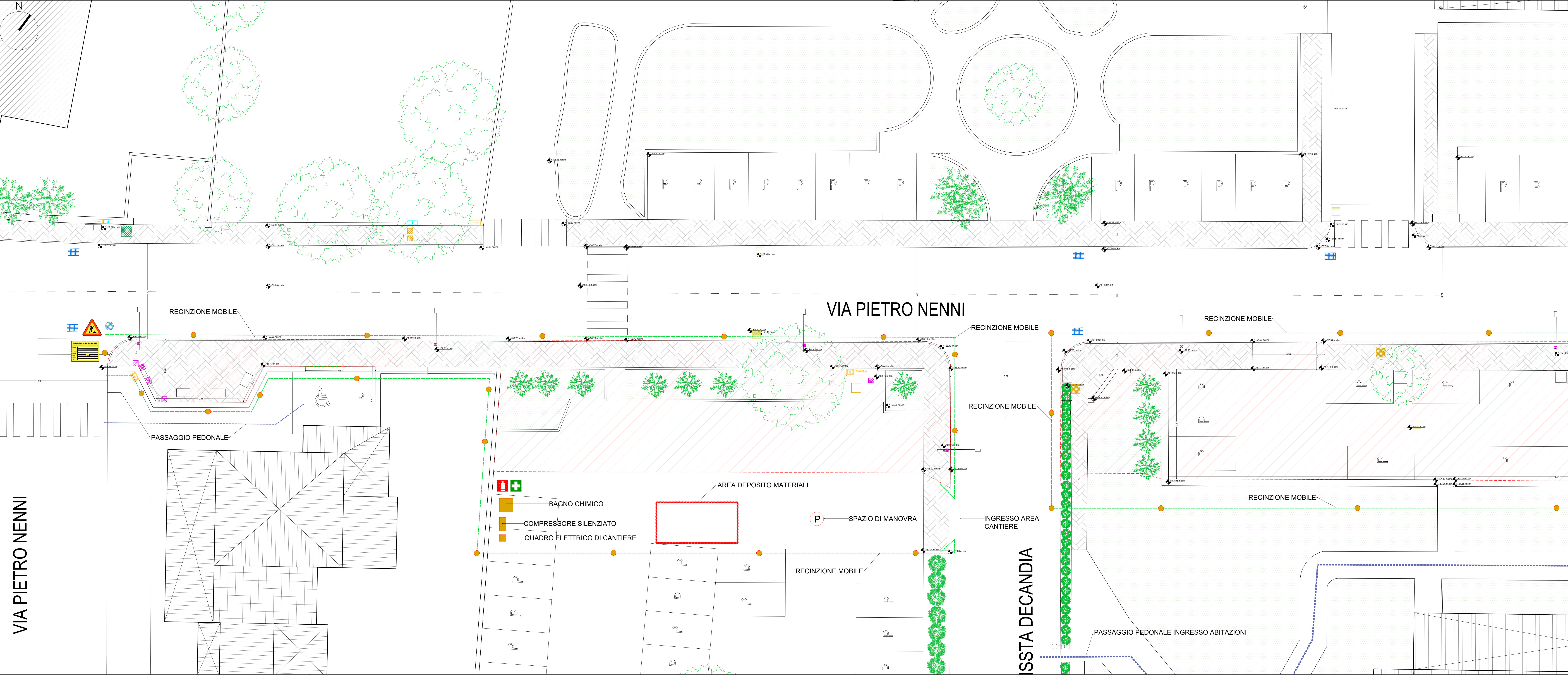
PLANIMETRIA DI CANTIERE - ZOOM AREA ALLESTIMENTO CANTIERE
