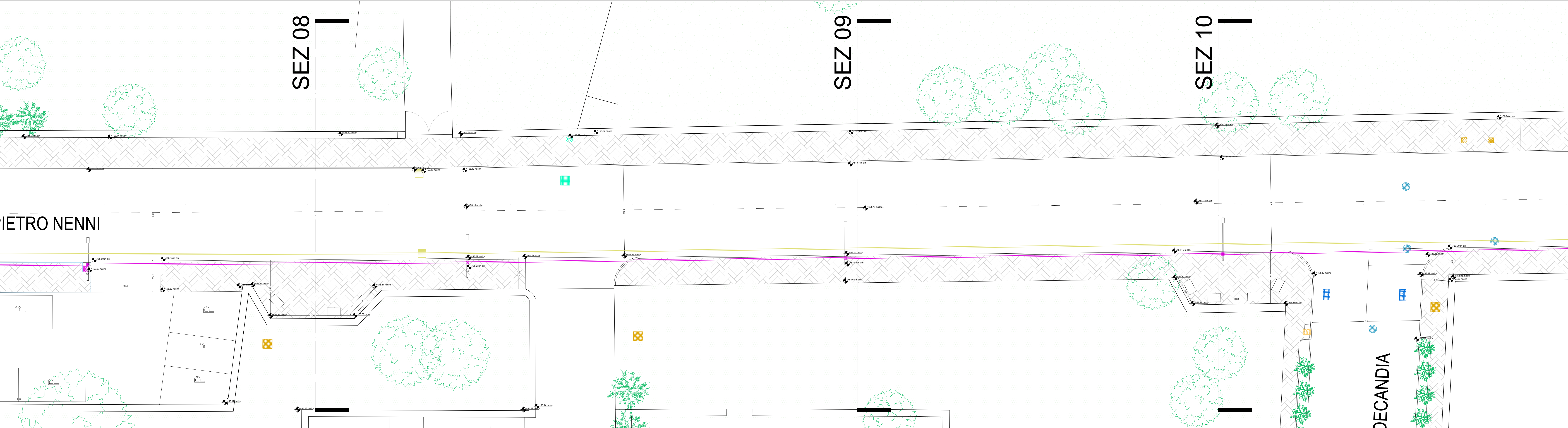
PLANIMETRIA STATO DI FATTO
