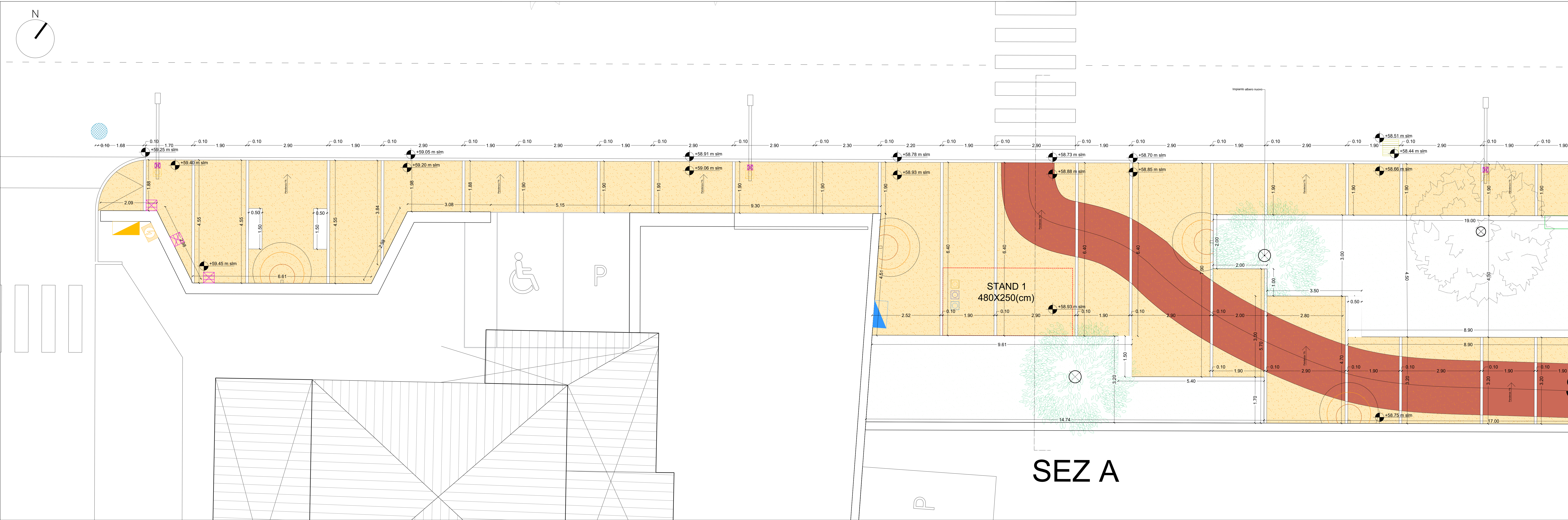
PLANIMETRIA ESECUTIVA
