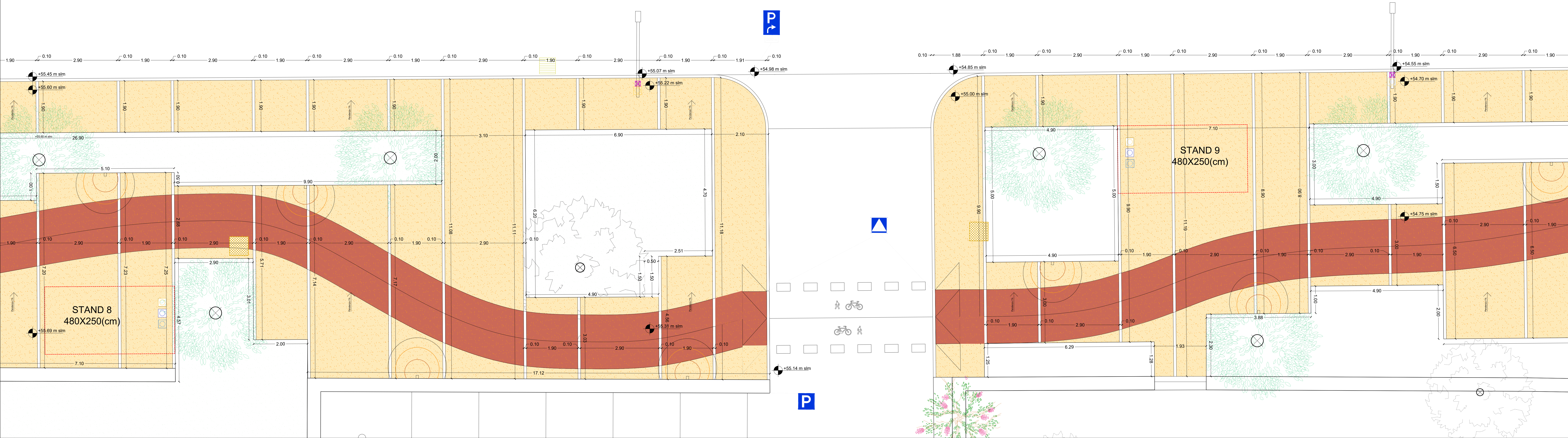
PLANIMETRIA ESECUTIVA
