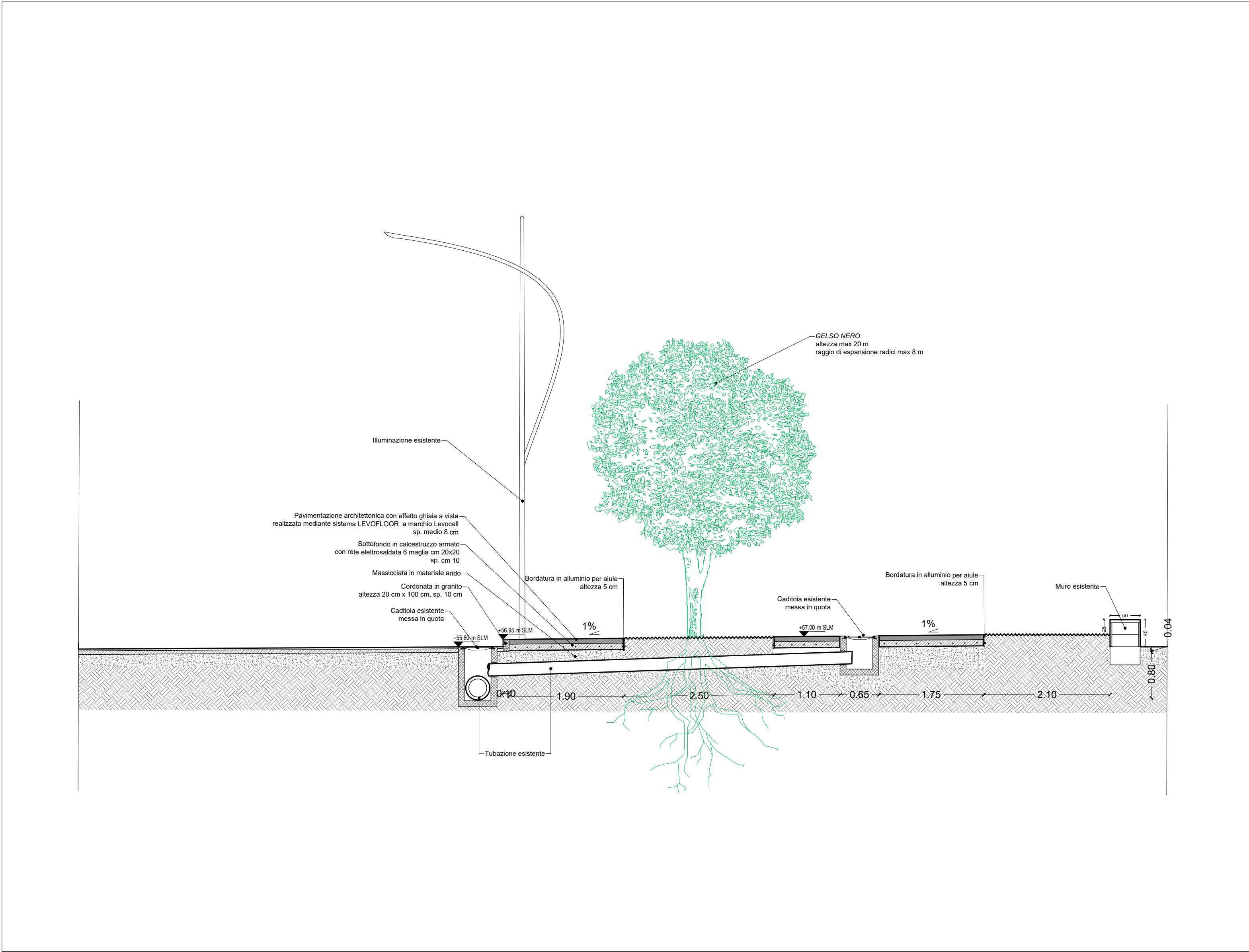
SEZIONE C
