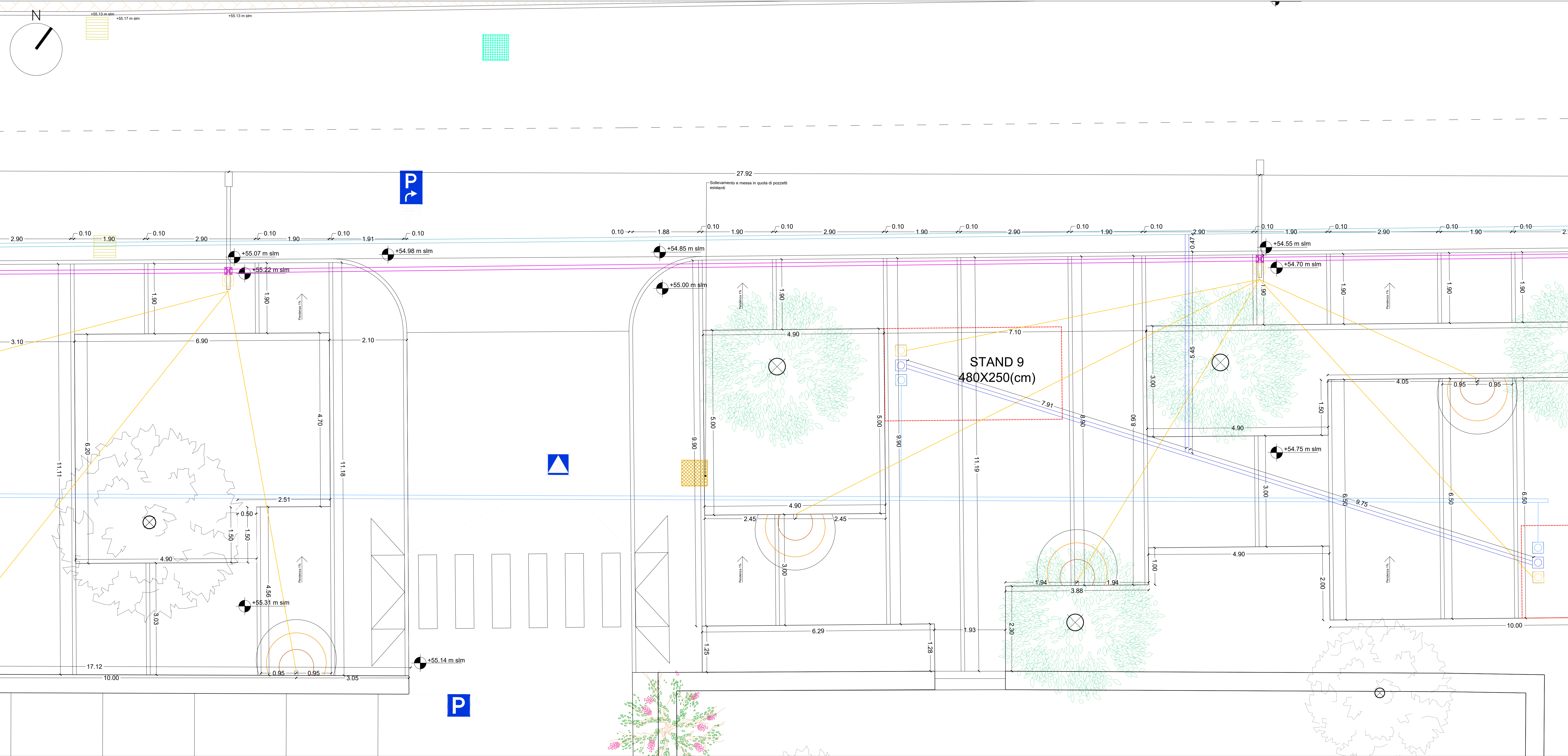
PLANIMETRIA ESECUTIVA - SOTTOSERVIZI
