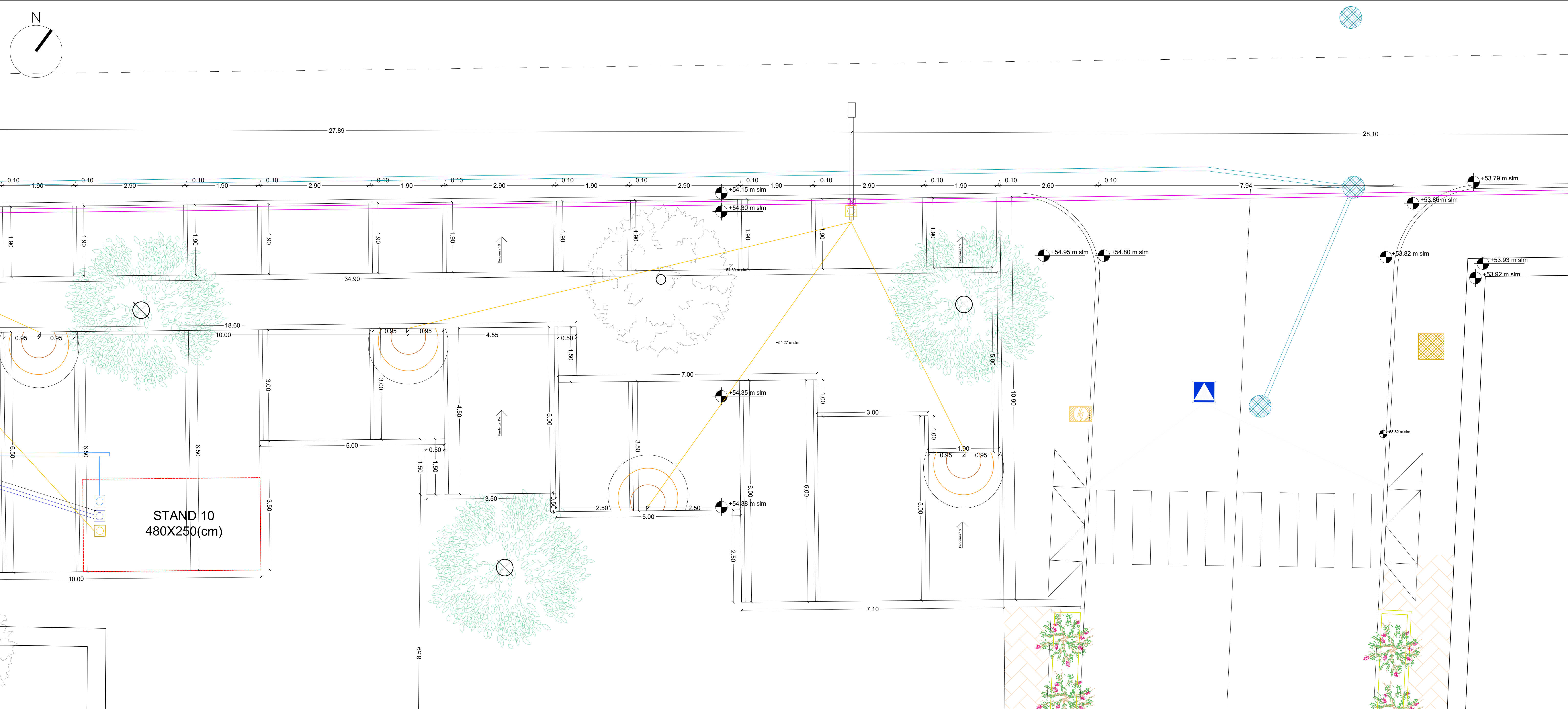
PLANIMETRIA ESECUTIVA - SOTTOSERVIZI
