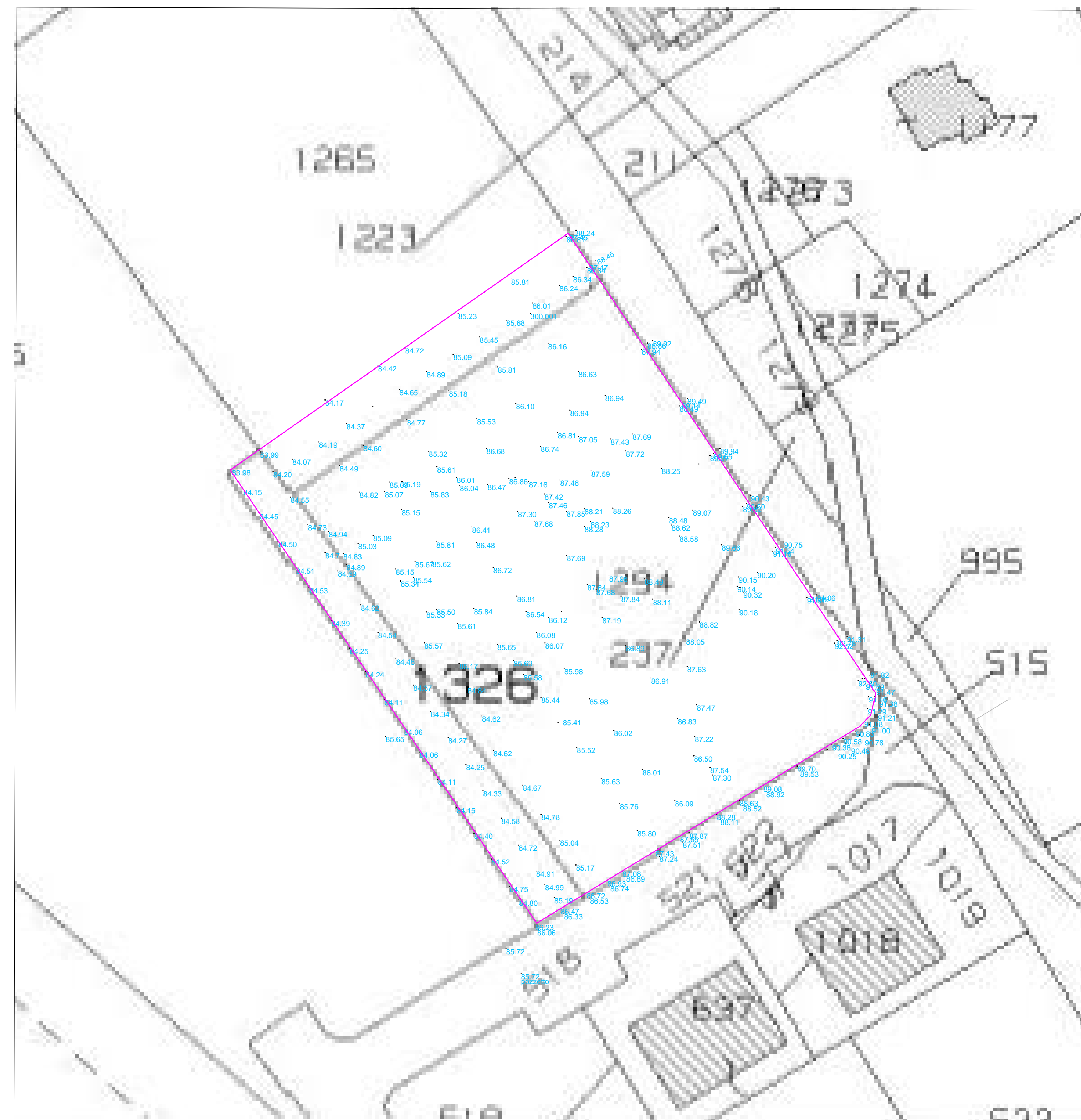
Ingrandimento catastale con sovrapposizione rilievo 1: 500
