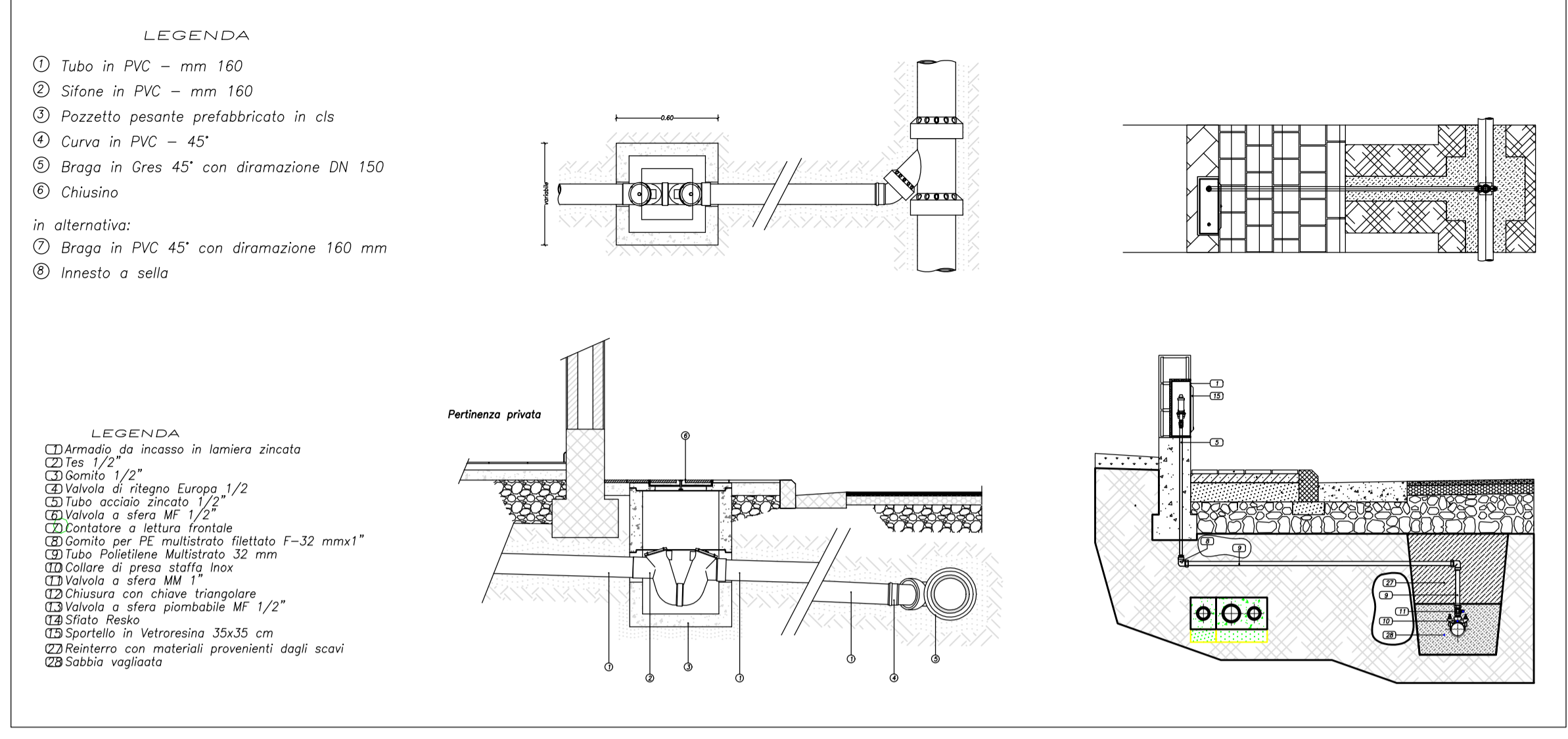
PARTICOLARI COSTRUTTIVI
